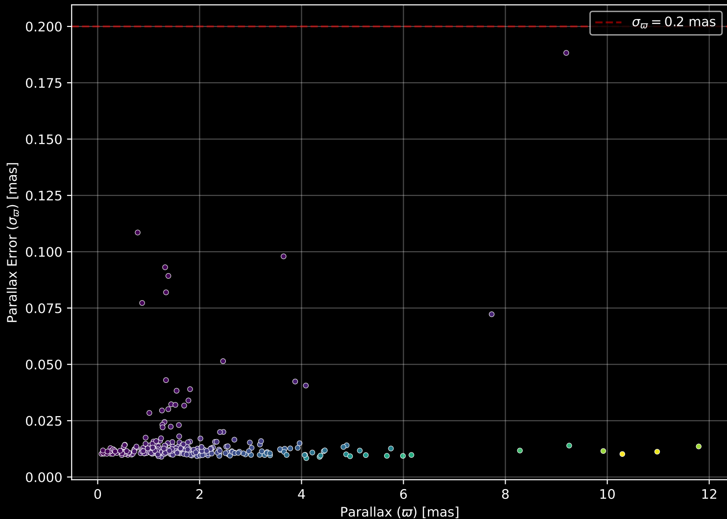
GALAH DR4 Field: [411] Parallax Quality (n= 287)
