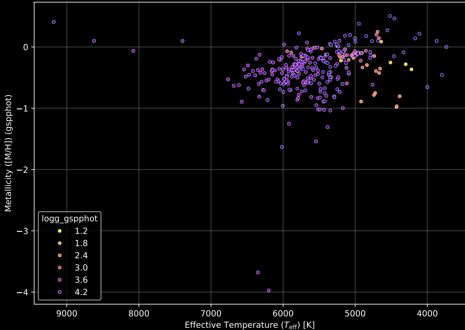
GALAH DR4 Field: [411] Stellar Population Parameters (n= 287)
